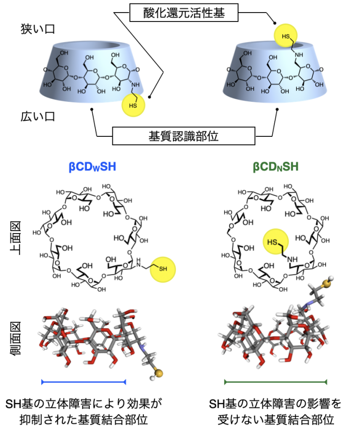
図 1 a) 「寛容的」な基質認識とタンパク質フォールディングのコンセプト図、b) 本研究で開発した人工フォールディング促進酵素 \beta\text{CD}_w\text{SH} 、およびその比較分子 \beta\text{CD}_n\text{SH} の分子構造
