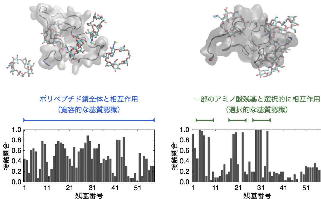
図2 分子動力学シミュレーションの結果
