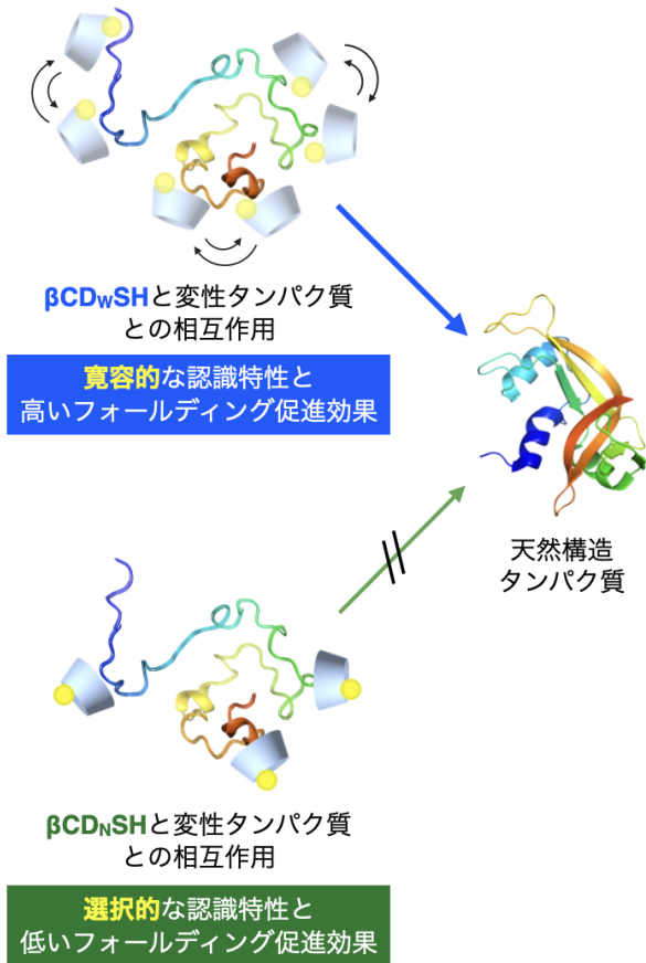
図 1 a) 「寛容的」な基質認識とタンパク質フォールディングのコンセプト図、b) 本研究で開発した人工フォールディング促進酵素 \beta\text{CD}_w\text{SH} 、およびその比較分子 \beta\text{CD}_n\text{SH} の分子構造
